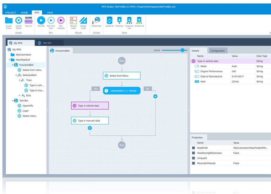
Tricentis RPA Studio: Modellbasierte Automatisierung mit Flow Chart
